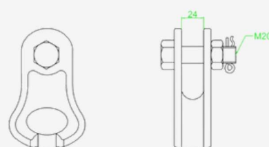
GUARDACABO HORQUILLA
